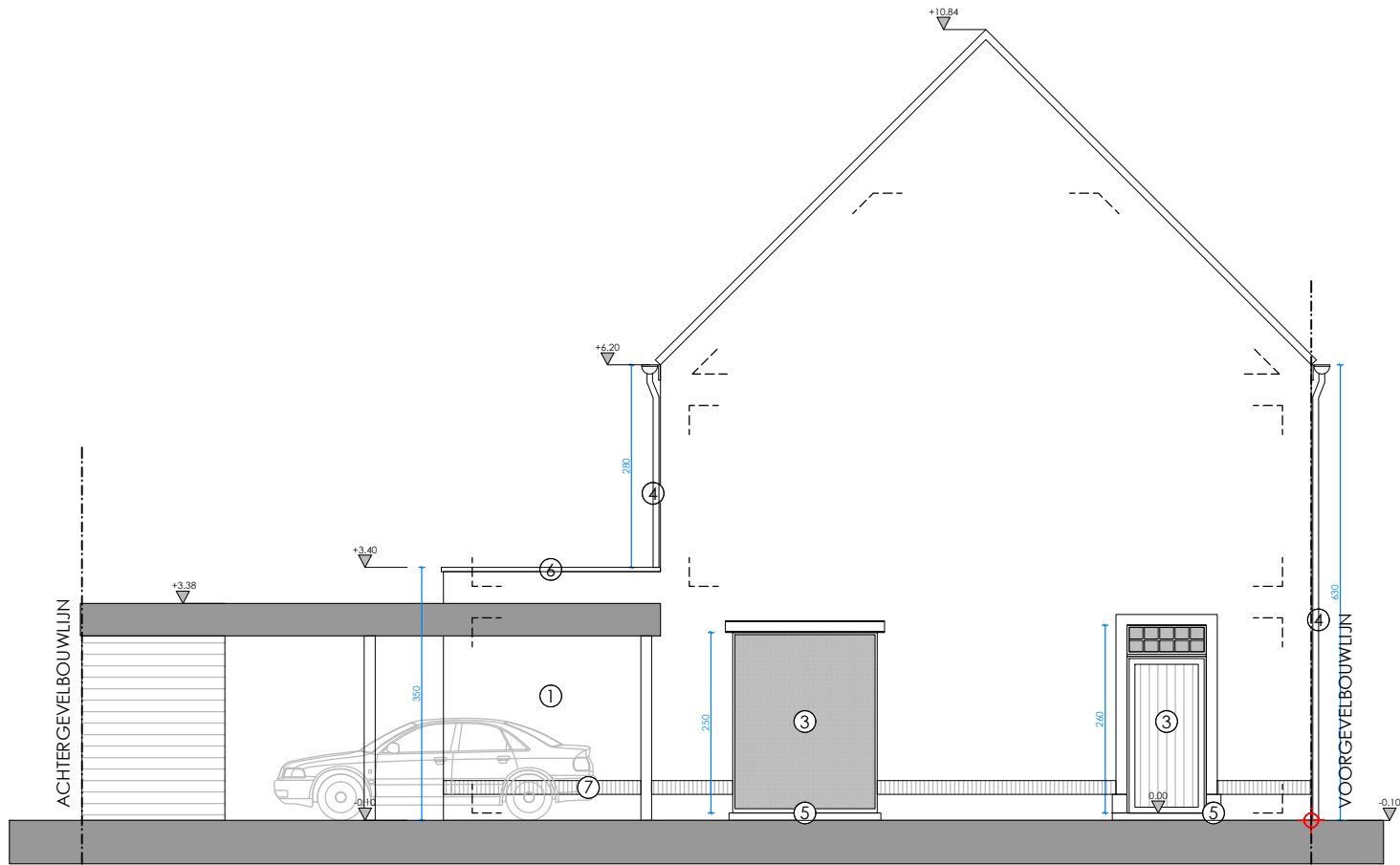
Zijgevel links
