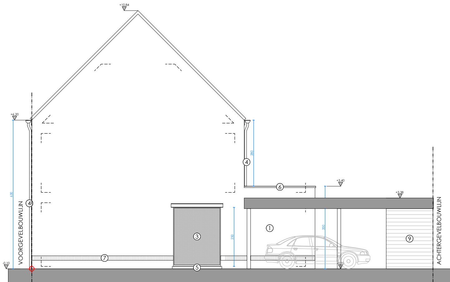
Zijgevel rechts
